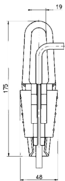
Держатель кабеля Артикул № 40/00061389
