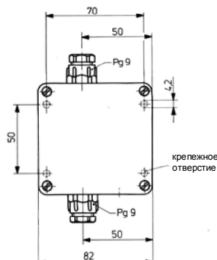
Клеммная коробка с компенсацией давления Артикул № 40/00061206
