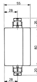
Клеммная коробка с компенсацией давления Артикул № 40/00061206
